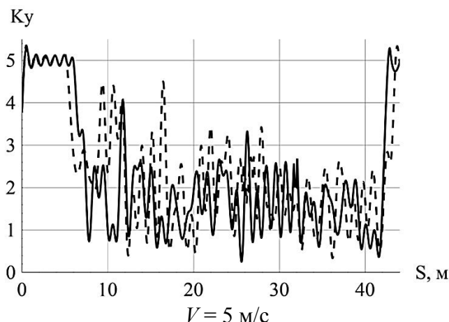
Рис. 6. Зависимость коэффициента запаса устойчивости при движении в кривой: -- набігаюче колесо з додатковою кінематичною подвижністю; — жорстко встановлене в вертикальній площині набігаюче колесо
